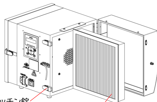
2次フィルター
