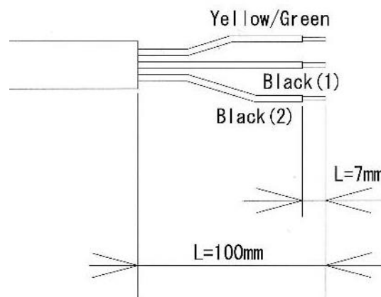
電源ケーブル 先端図
