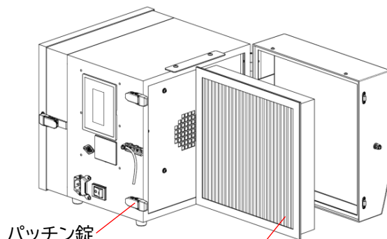
2次フィルター
