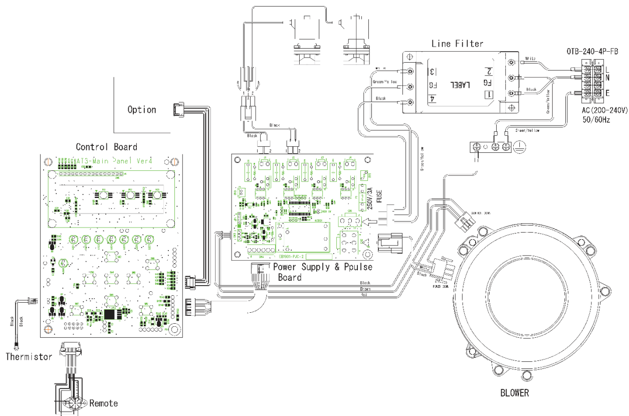
CHP-1600AT3
